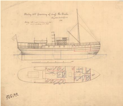
Ritning till ångfartyget Per Brahe 1889, Sjöhistoriska museet
