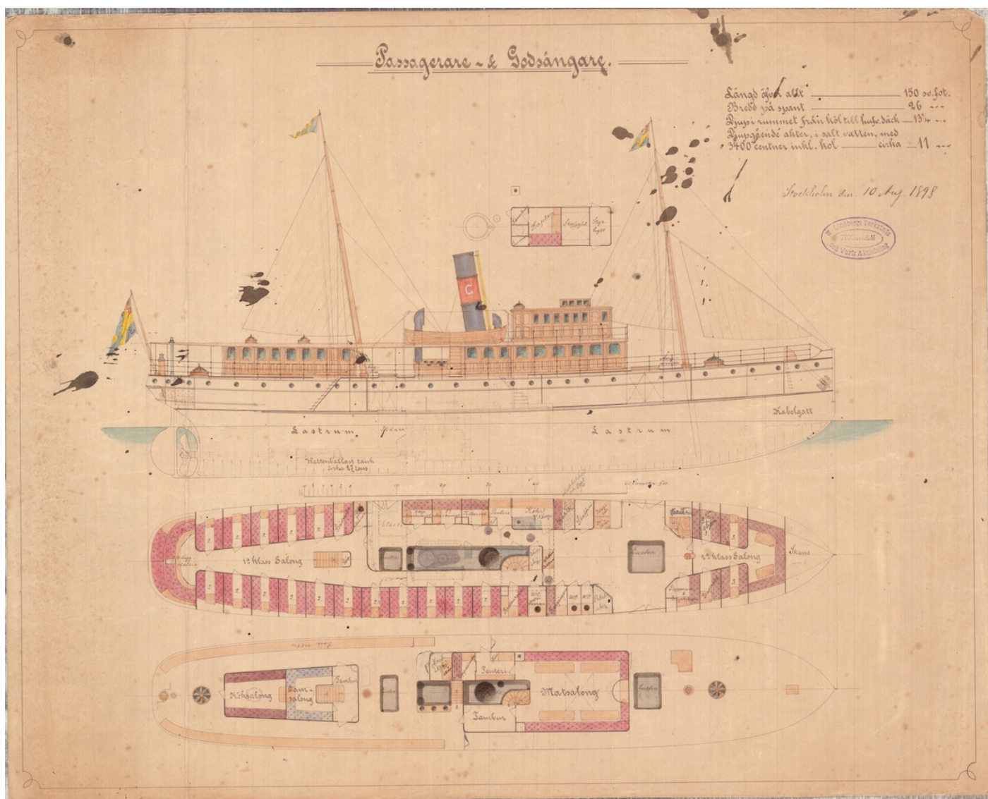
SR 2768. Ritning över S/S Hansa, byggd vid W. Lindbergs mekaniska verkstad.
